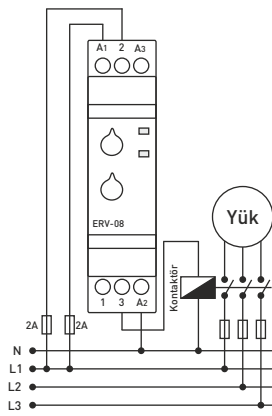
ERV-08 için Bağlantı Şeması
