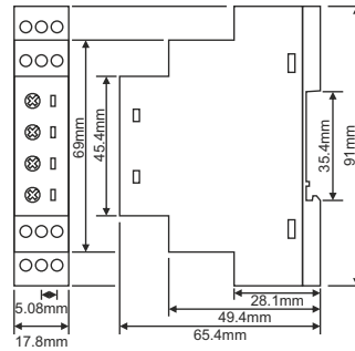
ERV-08 için Boyutlar
