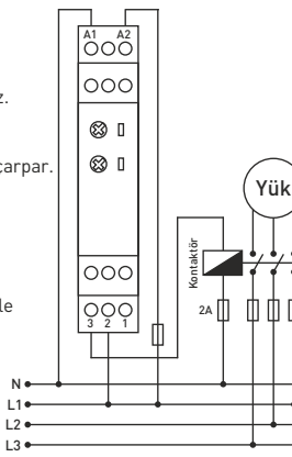
ERV-08M için Bağlantı Şeması
