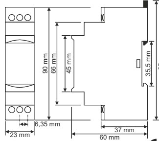
ERV-08 için Boyutlar
